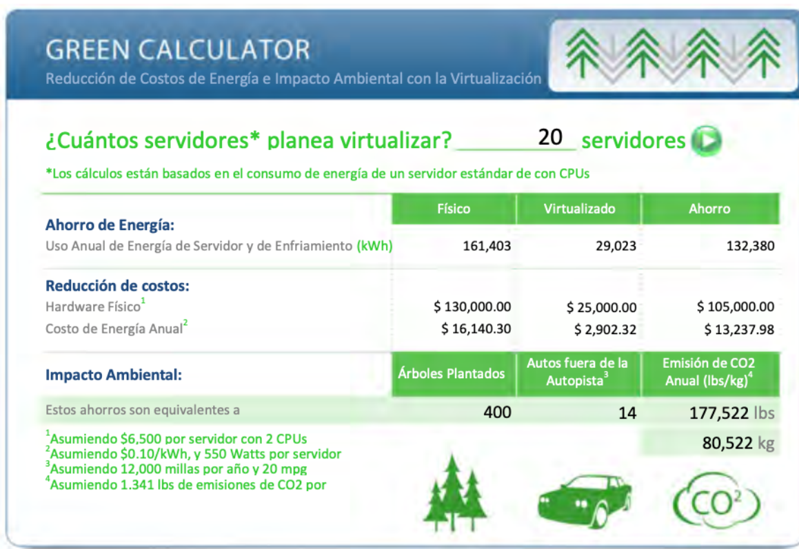
Figura 2.1. Resultados de la herramienta Green Calculator de VMware considerando la virtualización de 20 servidores.
